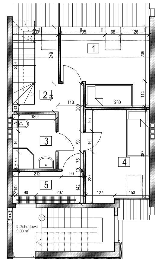
Rzut antresoli
