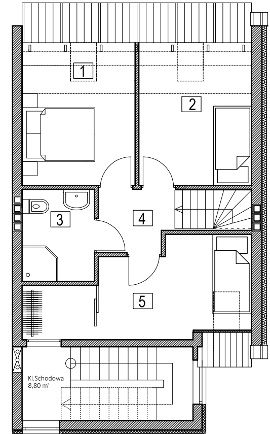
Rzut antresoli
